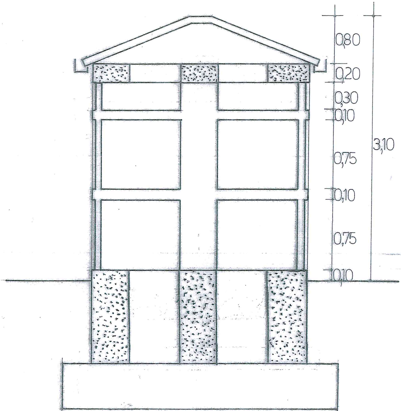
SEZIONE A-A
