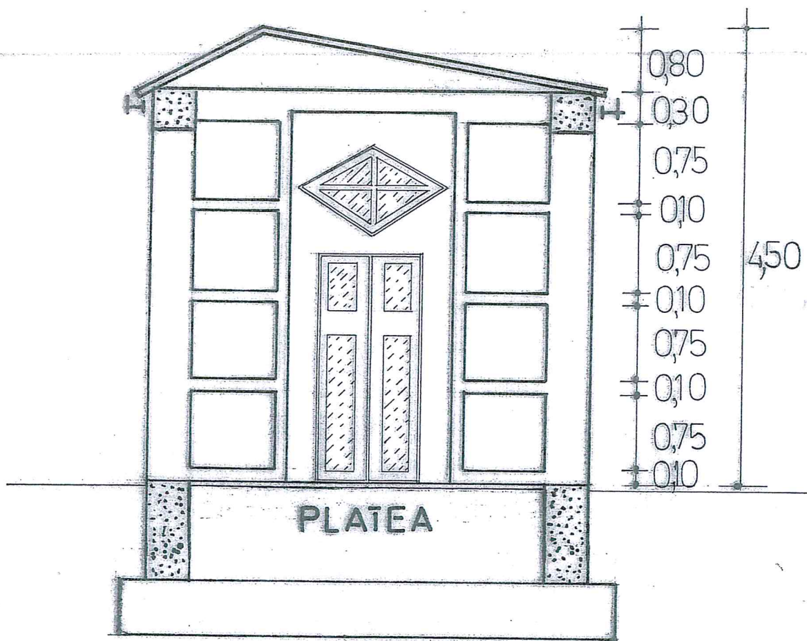
SEZIONE A'-A
